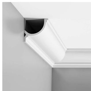
C902 ORAC モールディング 海外取寄品 税抜価格(個)：¥11,000 価格(ケース)：¥132,000 素材：Purotouch (高密度ポリウレタン) サイズ(cm)：200 x 10.3 x 10.3 種類：コーニス(廻り縁) 機能：ライティング
