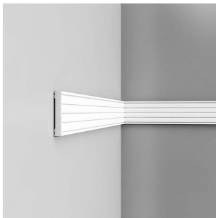
P5020 ORAC モールディング 海外取寄品 税抜価格(個)：¥7,100 価格(ケース)：¥113,600 素材：Purotouch (高密度ポリウレタン) サイズ(cm)：200 x 9.1 x 1.3 種類：パネル(腰壁) 機能：-
