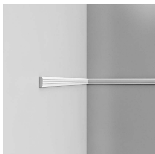
P5021F ORAC モールドイング 海外取寄品 税抜価格(個): ¥6,700 価格(ケース): ¥335,000 素材: Purotouch (高密度ポリウレタン) サイズ(cm): 200 x 3.1 x 0.9 種類: パネル(腰壁) 機能: フレックス(R対応) R寸法(cm) 前後方向/上下方向: 20 / 70
