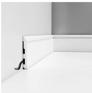
SX118 ORAC モールディング 海外取寄品 税抜価格(個)：¥4,900 価格(ケース)：¥58,800 素材：Duropolymer (高密度ポリスチレン&ポリマー) サイズ(cm)：200 x 13.8 x 1.8 種類：スカーディング(巾木) 機能：-
